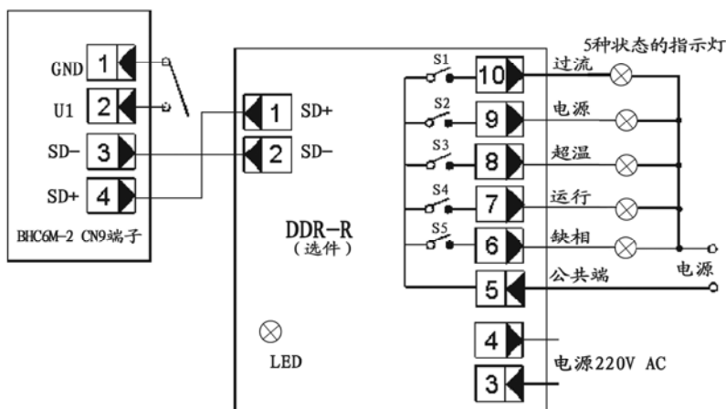
图 2-3 DDR-R 接线图
